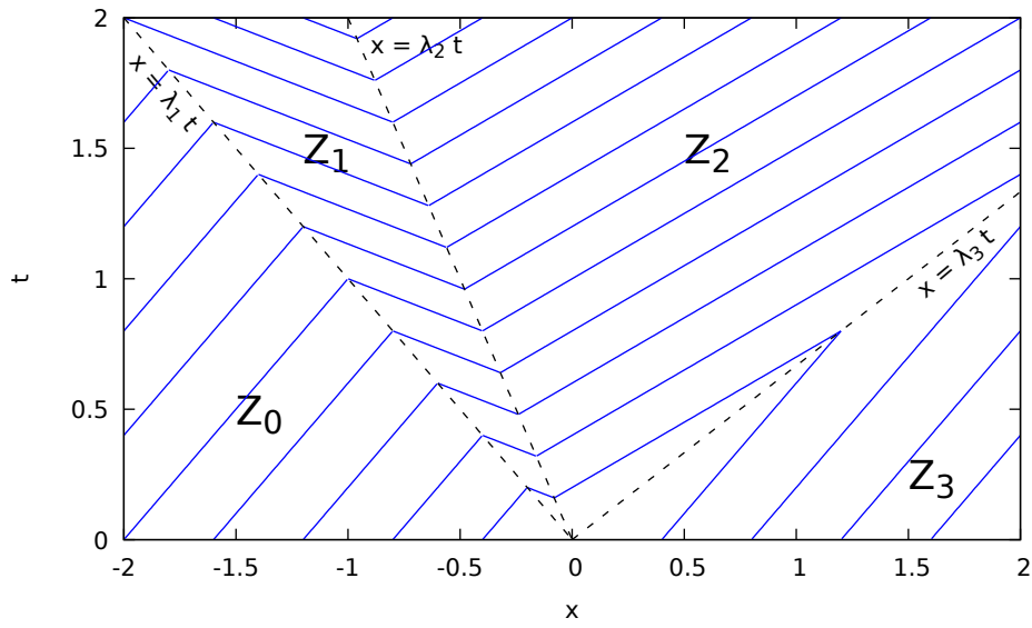
FIGURE 8 – Droites caractéristiques dans le cas d’une solution faible avec N = 3 . Les paramètres \lambda_1 et \lambda_3 peuvent être choisis librement (en respectant la contrainte \lambda_1 < a < \lambda_3 ) pour construire d’autres solutions faibles.
