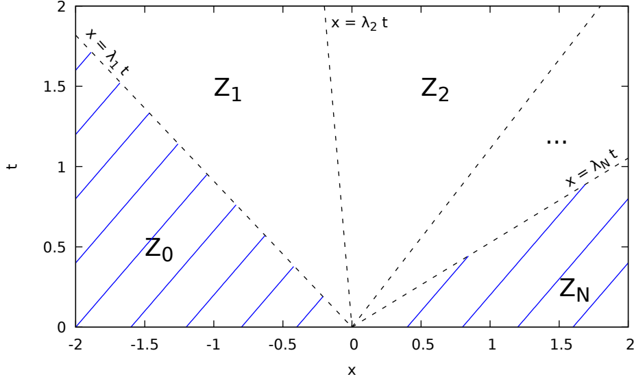
FIGURE 7 – Non unicité des solutions faibles constantes par morceaux. Les limites entre zones sont représentées par des lignes pointillées noires; les droites caractéristiques sont tracées en bleu (ici dans un cas où a > 0 ).
